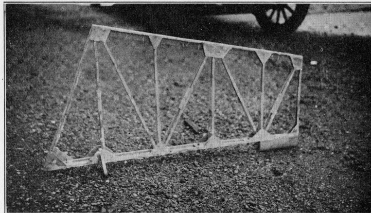
Plate XXX. Prüfling Rudder
